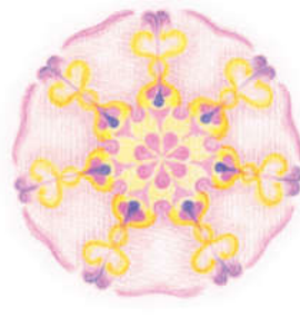
15-01 Mond Merkur
