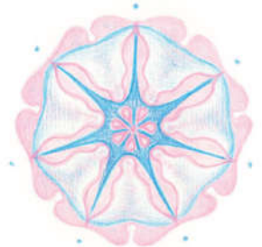
13-01 Sonne Saturn
