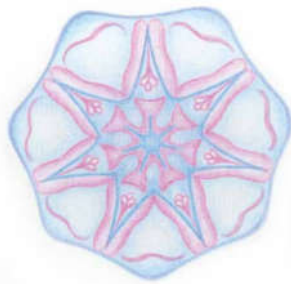
18-01 Mond Saturn
