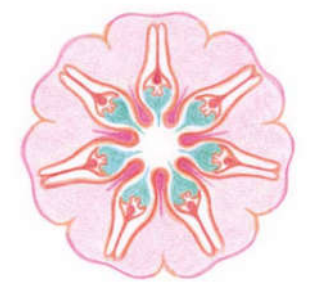
21-02 Mars Venus
