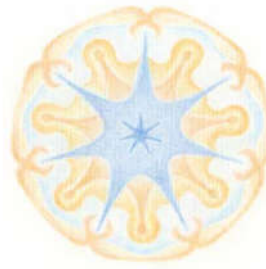
27-01 Jupiter Saturn
