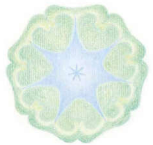
28-01 Venus Saturn
