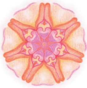
14-01 Mond Mars
