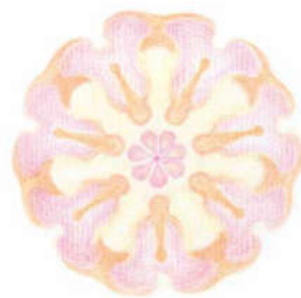
11-01 Sonne Jupiter
