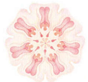
9-02 Sonne Mars
