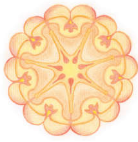
20-03 Mars Jupiter
