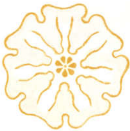
7-01 Sonne
