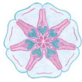
17-04 Mond Venus
