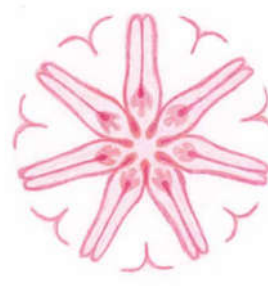
5-03 Mars
