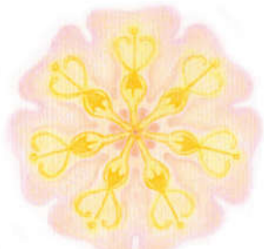
10-02 Sonne Merkur
