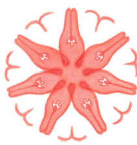
5-02 Mars
