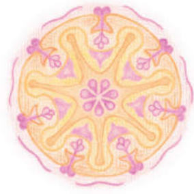
16-02 Mond Jupiter
