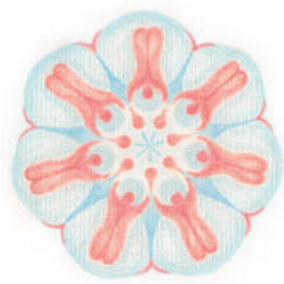
22-01 Mars Saturn
