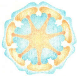
26-01 Jupiter Venus
