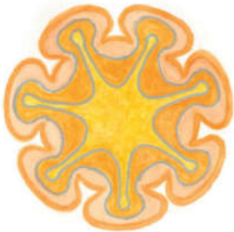
3-03 Jupiter
