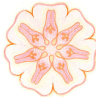
9-01 Sonne Mars
